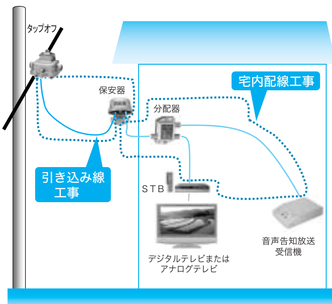
引き込み線工事と宅内配線工事
